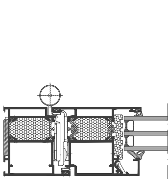
Horizontalschnitt
