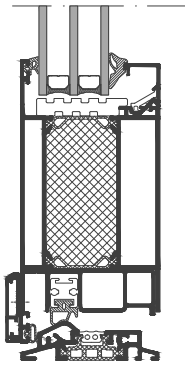
Vertikalschnitt
