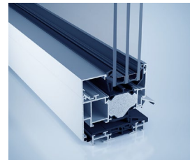
Barrierefrei heroal W 77 UD
