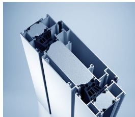
Lüftungsklappe heroal W 72 VF
