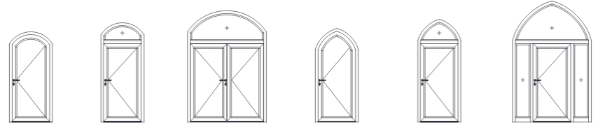
Ein- und zweiflügelige Formelemente
